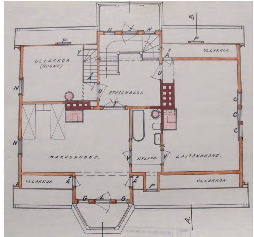
Ullakkokerroksen pohjapiirros.
