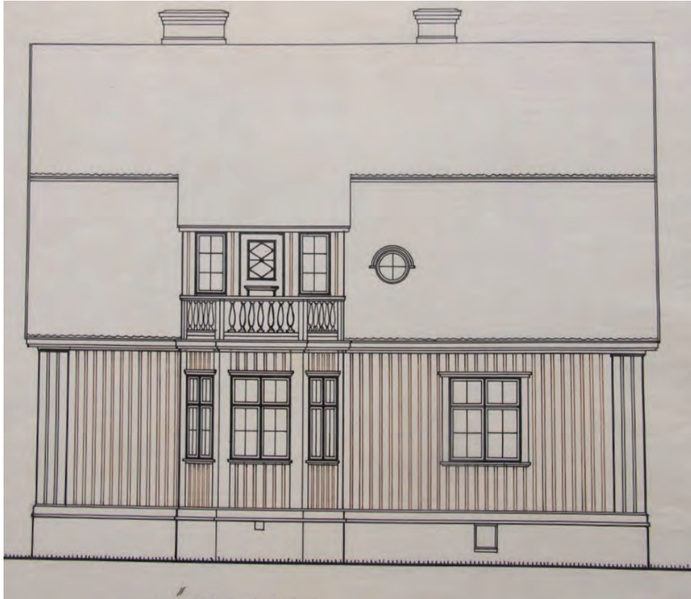
Julkisivu pohjoiseen.
