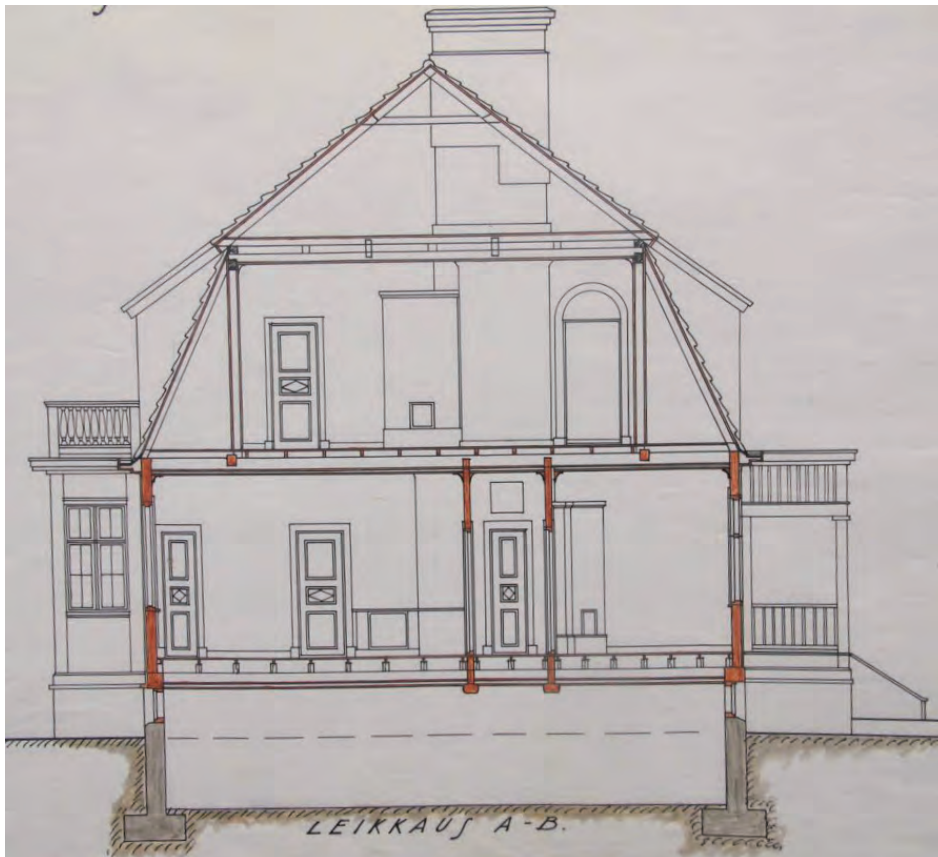
Leikkaus.
